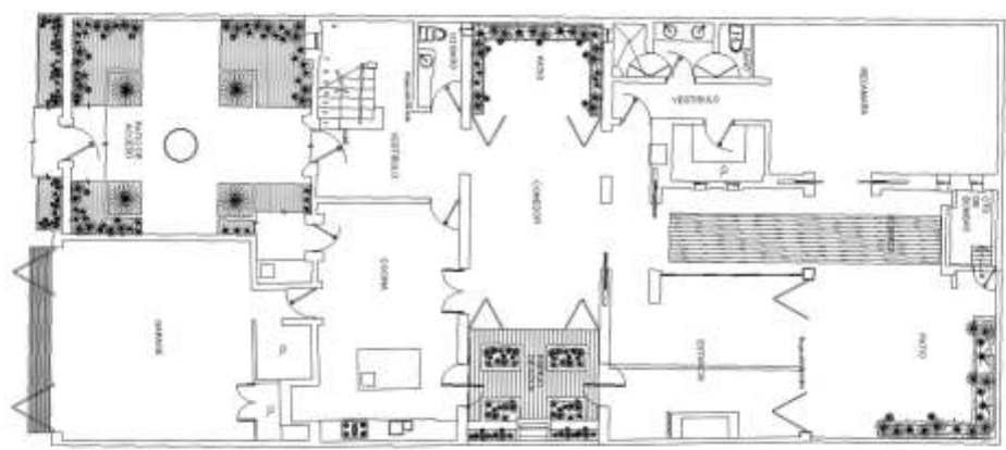
PLANTA BAJA | FIRST FLOOR
