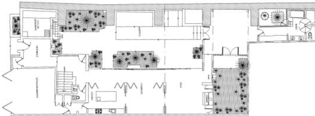
PLANTA BAJA | FIRST FLOOR
